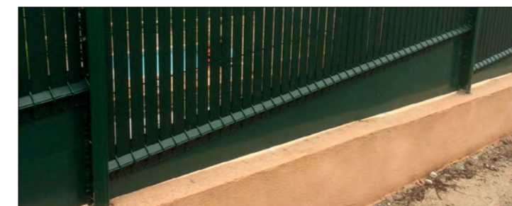
Tôle de soubassement "spécial pente" fabriquée sur-mesure
